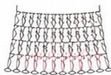
dodawanie ściegów
